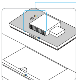
Fig. 1 Inseste in versione standard con stick (1) all'interno della cappa e pannello di controllo (2) La cappa viene controllata tramite l'interruttore principale del piano cottura (3) o il pannello di controllo della cappa. La temperatura del colore è di 4.000 K.
