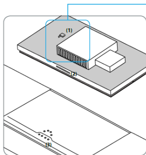
Afb. 1 Afzuigkap in standaarduitvoering met Stick (1) in de kap en bedieningspaneel (2) De kap wordt bediend via de hoofdschakelaar op de kookplaat (3) of het bedieningspaneel van de kap. De kleurtemperatuur is 4.000 K.
