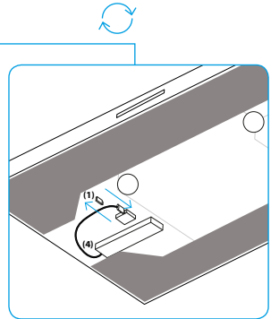
Abb. 3 Einfache Montage des Receivers Der Receiver lässt sich ohne zusätzliches Werkzeug einfach montieren: Fettpfänger an der Unterseite der Haube abnehmen, Stick (1) im Inneren der Haube entfernen und den Receiver (4) einstecken.
