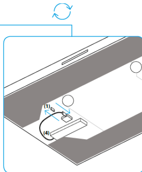
Fig. 3 Montaggio semplificato del ricevitore Il ricevitore può essere facilmente installato senza attrezzature aggiuntive: Rimuovere il filtro di grasso sul lato inferiore della cappa, rimuovere il bastone (1) all'interno della cappa e inserire il ricevitore (4).
