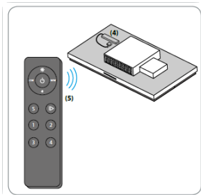
Fig. 4 Collegare il ricevitore (4) e il telecomando opzionale (5): 1. Rimuovere la pellicola protettiva dalla batteria 2. Per impostare il telecomando, tenere premuto 10 secondi la Learning Key sul ricevitore (4) 3. Premere per breve tempo la Learning Key sul ricevitore (4) e selezionare direttamente la zona desiderata (1 2 3 4) sul telecomando 4. Le luci LED lampeggiano una volta - il ricevitore è connesso 5. Per spegnere la Learning Key sul ricevitore (4) premere 10 secondi
