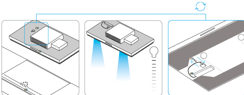
Fig. 1 Köksfläkt i standardutförande med stift (1) inne i spiskåpan och styrpanel (2) Spiskåpan styrs med huvudströmbrytaren på spishällen (3) eller med spiskåpan styrpanel. Färgtemperaturen är 4.000 K.
