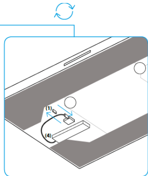
Afb.3 Eenvoudige montage van de ontvanger De ontvanger is eenvoudig te installeren, zonder extra gereedschap. Verwijder het vetfilter uit de onderkant, verwijder de stick (1) uit de binnenzijde van de kap en plaats de ontvanger (4).
