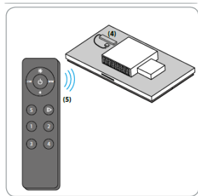
Afb.4 Koppelen van de ontvanger (4) en optionele afstandsbediening (5)
