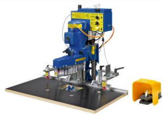
BlueMax Mini Modular mit 6- Spindelbohrgetriebe für Verbinder und Scharniere. Foto: Hettich
